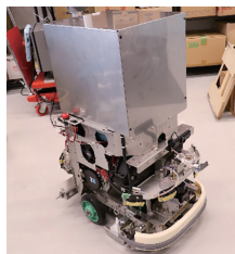
自律移動ロボット
