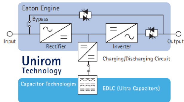
↑ 瞬時電圧低下保護装置（SRT）
