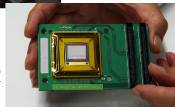
機関部品となる MEMS デジタル・マイクロミラー
